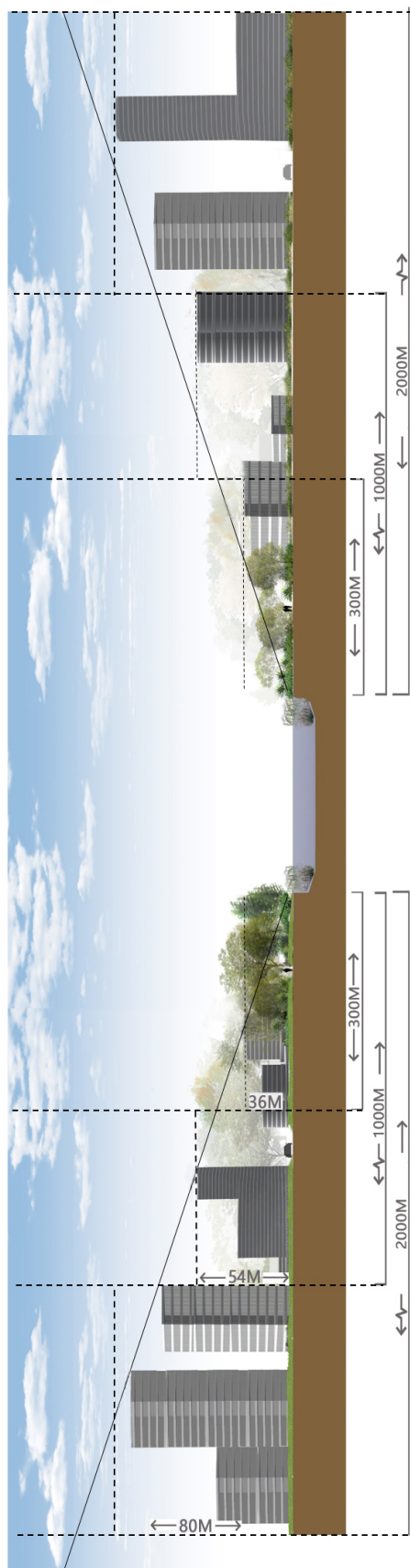
附图4 城镇发展区老城改造范围限高剖面示意图
